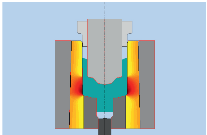
Wirkende Kräfte am Werkzeug
